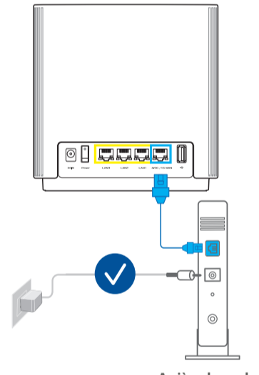
Arrière du modem
